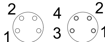
孔母头 针公头
